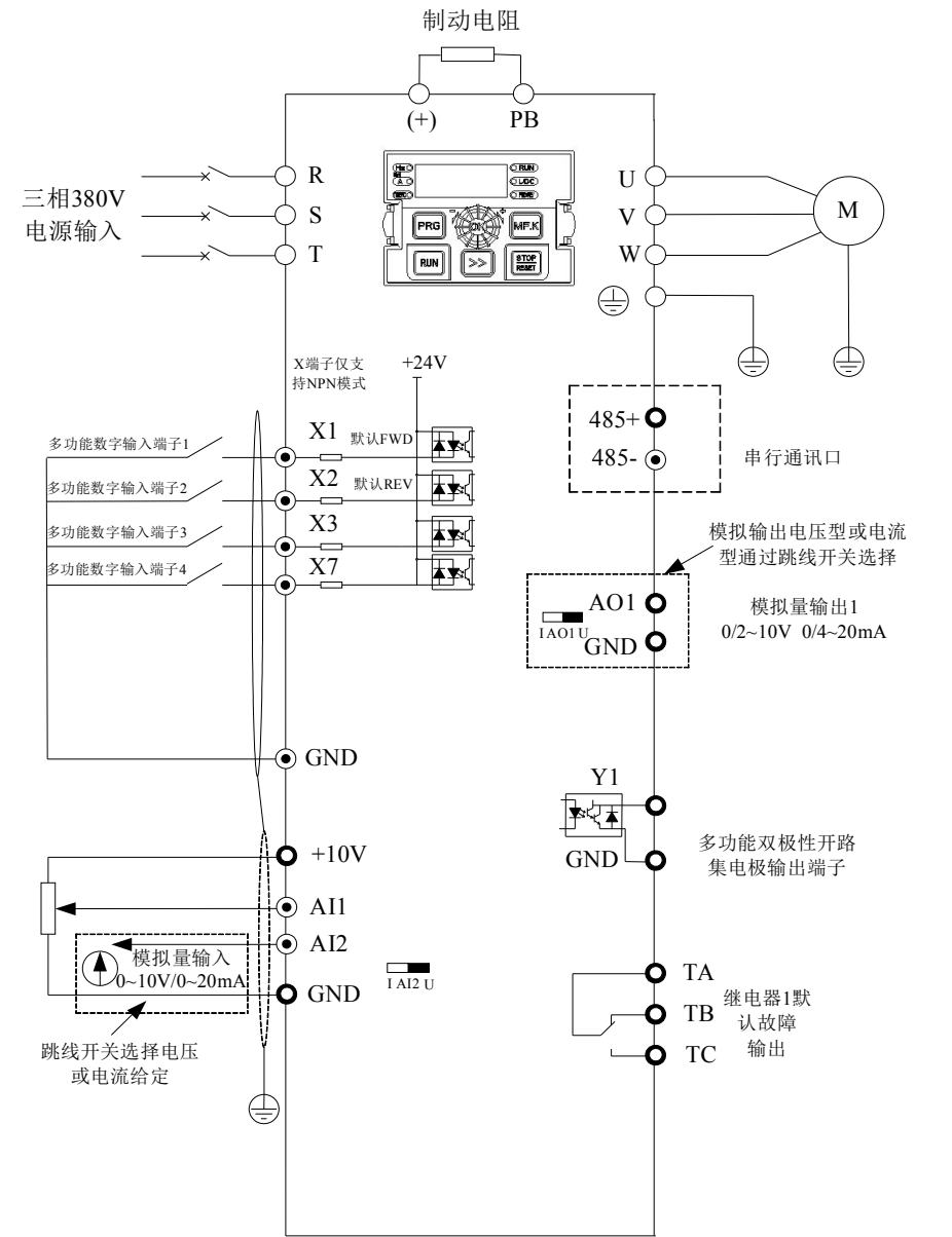
图3-1. 三相380V 2.2kW (4T:380V) 及单相220V (2S) 2.2kW(输入接L N或R T)以下变频器接线图 备注：数字输入端子X 2.2kW 以下仅支持内部供电 NPN 模式（即 X 短接 COM 有效）。AI2, AO1 跳线开关出厂默认电压模式。
