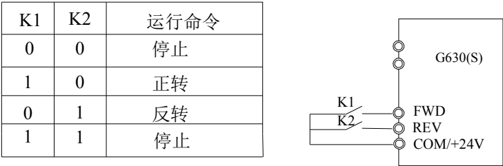
图 3-13. 两线式运转模式 1
