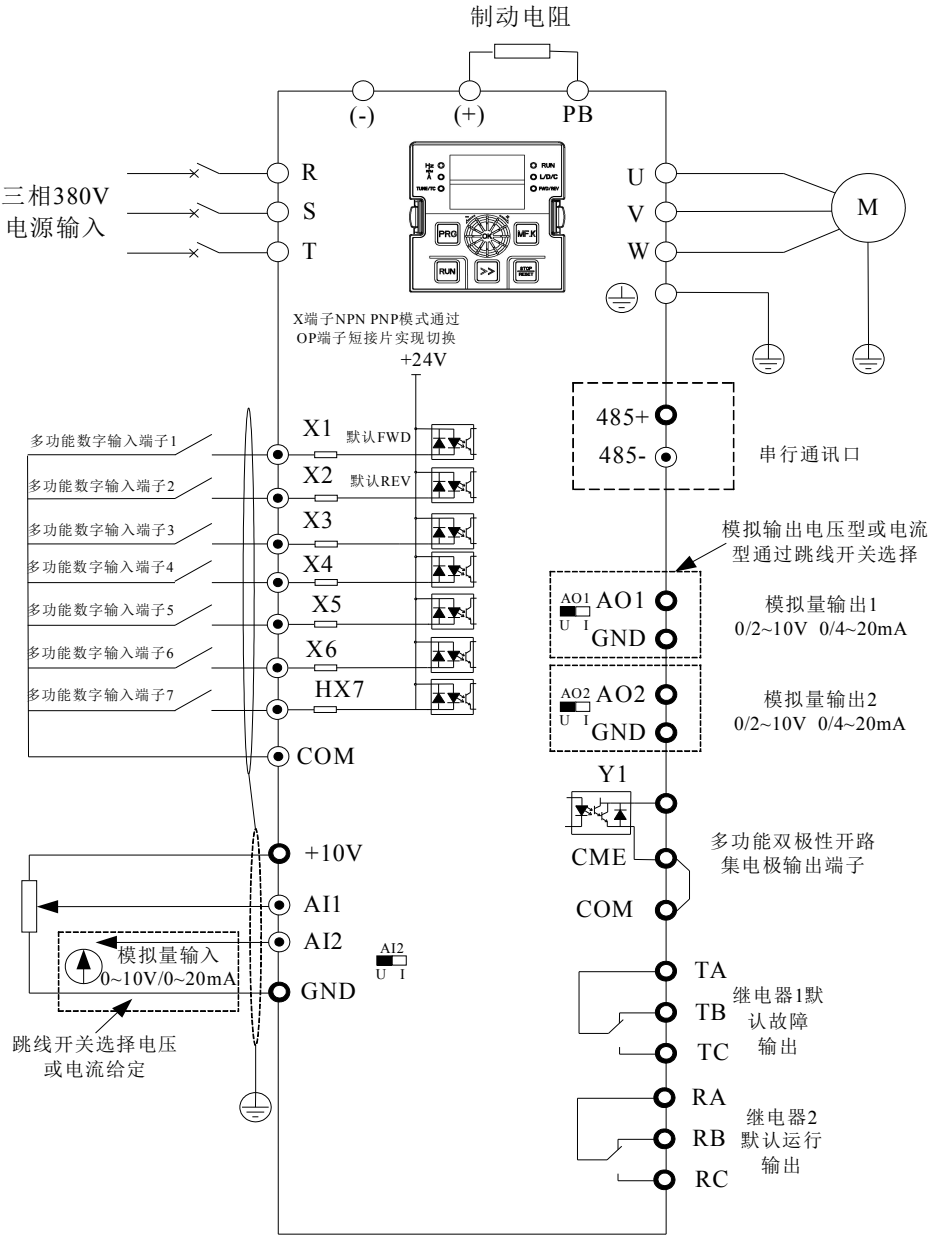
图 3-2. 三相 380V 4.0~ 30kW (4T:380V) 及单相 220V (2S) 5.5kW 以下(输入接 R T)变频器接线图 备注：数字输入端子 X 跳线开关出厂默认（OP 端子连接 24V 端子）NPN 模式（即 X 短接 COM 有效）， AI2, AO1, AO2 跳线开关出厂默认电压模式。
