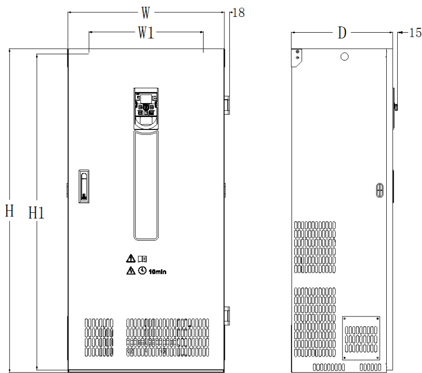
图 2-6. 380V 220kW 以上变频器外型尺寸及安装尺寸示意图
