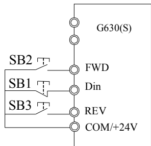
图 3-15. 三线式运转模式 1
