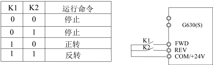
图3-14. 两线式运转模式2
