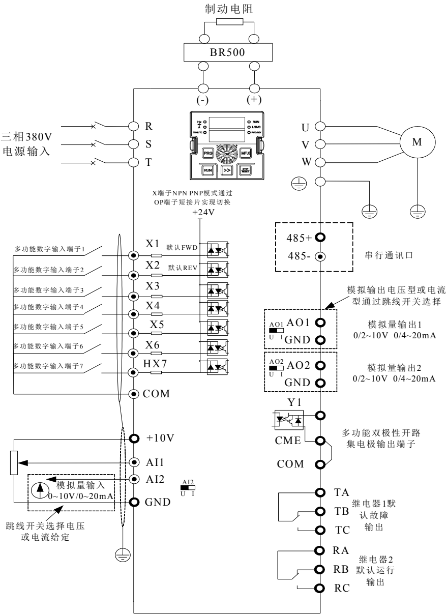
图 3-3. 三相 380V 37 ~ 75 kW (4T:380V) 变频器不带制动单元功能接线图 备注：数字输入端子 X 跳线开关出厂默认（OP 端子连接 24V 端子）NPN 模式（即 X 短接 COM 有效），AI2, AO1, AO2 跳线开关出厂默认电压模式。G630/G630S 系列 37~110kW 制动单元部分属选配功能，如有需求，订货时请说明，选配了制动单元功能的接线图参考图 3-2。
