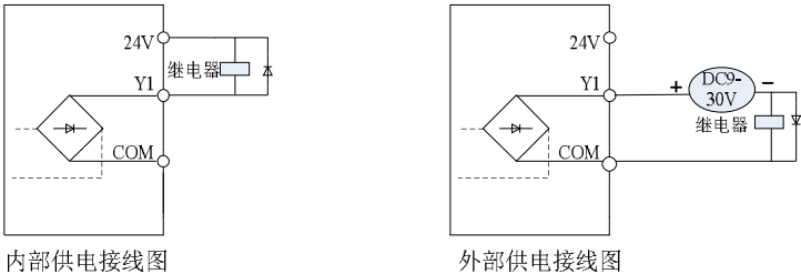
图 3-12. 数字输出端子Y1 接线示意图
