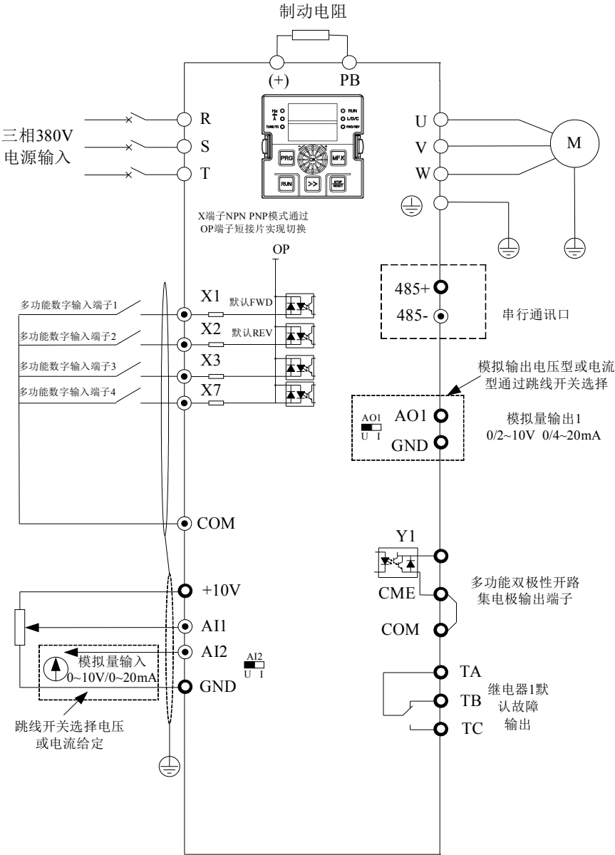
图3-1. 三相380V 2.2kW（4T:380V）及单相220V（2S）2.2kW(输入接L N或R T)以下变频器接线图 备注：数字输入端子X跳线开关出厂默认（OP端子连接24V端子）NPN模式（即X短接COM有效），PNP模式为选配功能，三相380V 2.2 kW及单相220V 1.5 kW以下如需选配PNP模式，订货时请说明。AI2,A01跳线开关出厂默认电压模式。
