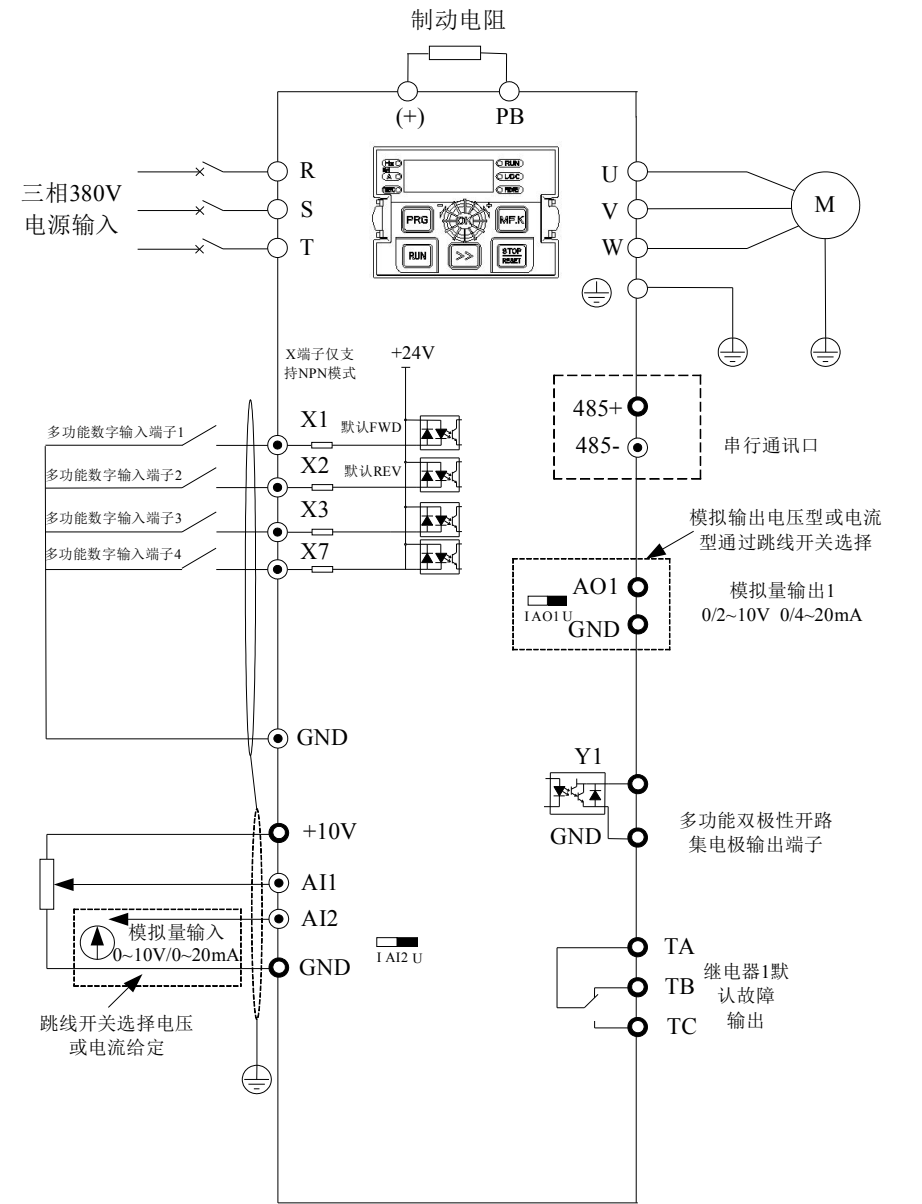
图3-1. 三相380V 2.2kW（4T:380V）及单相220V（2S）2.2kW(输入接L N或R T)以下变频器接线图 备注：数字输入端子X 2.2kW 以下仅支持内部供电 NPN 模式（即 X 短接 GND 有效）。AI2, AO1 跳线开关出厂默认电压模式。
