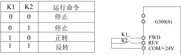
图3-14. 两线式运转模式2
