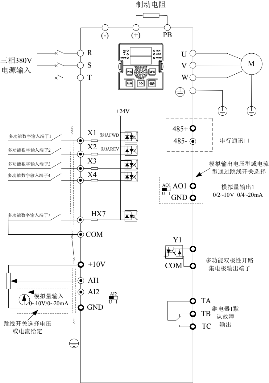
图 3-2. 三相 380V 4.0~ 30kW (4T:380V) 及单相 220V (2S) 5.5kW 以下(输入接 R T)变频器接线图 备注: 数字输入端子 X OP 端子短接 24V 出厂默认 NPN 模式(即 X 短接 COM 有效), AI2, AO1 跳线开关 出厂默认电压模式。
