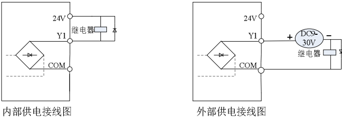
图 3-12. 数字输出端子Y1 驱动外接继电器接线示意图
