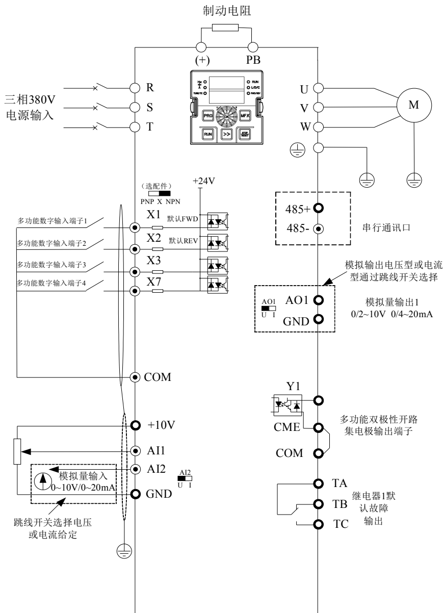
图3-1. 三相380V 2.2kW (4T:380V) 及单相220V (2S) 1.5kW(输入接L N或R T) 以下变频器接线图
