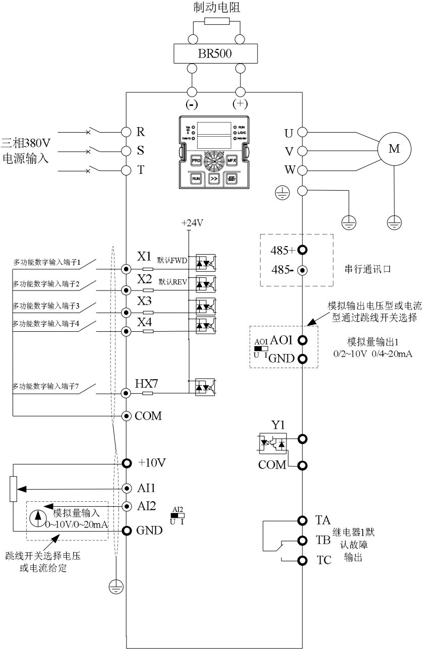
图 3-3. 三相 380V 37 ~ 75 kW (4T:380V) 变频器不带制动单元功能接线图 备注：数字输入端子 X OP 端子短接 24V 出厂默认 NPN 模式（即 X 短接 COM 有效），AI2, AO1 跳线开关出厂默认电压模式。G610/G610S 系列 37~110kW 制动单元部分属选配功能，如有需求，订货时请说明，选配了制动单元功能的接线图参考图 3-2。
