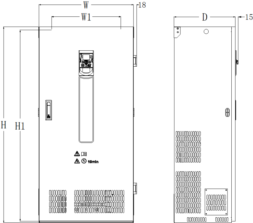
图 2-6. 160KW 以上变频器外型尺寸及安装尺寸示意图 表 2-2 G630/G630S 外形尺寸及安装孔位尺寸
