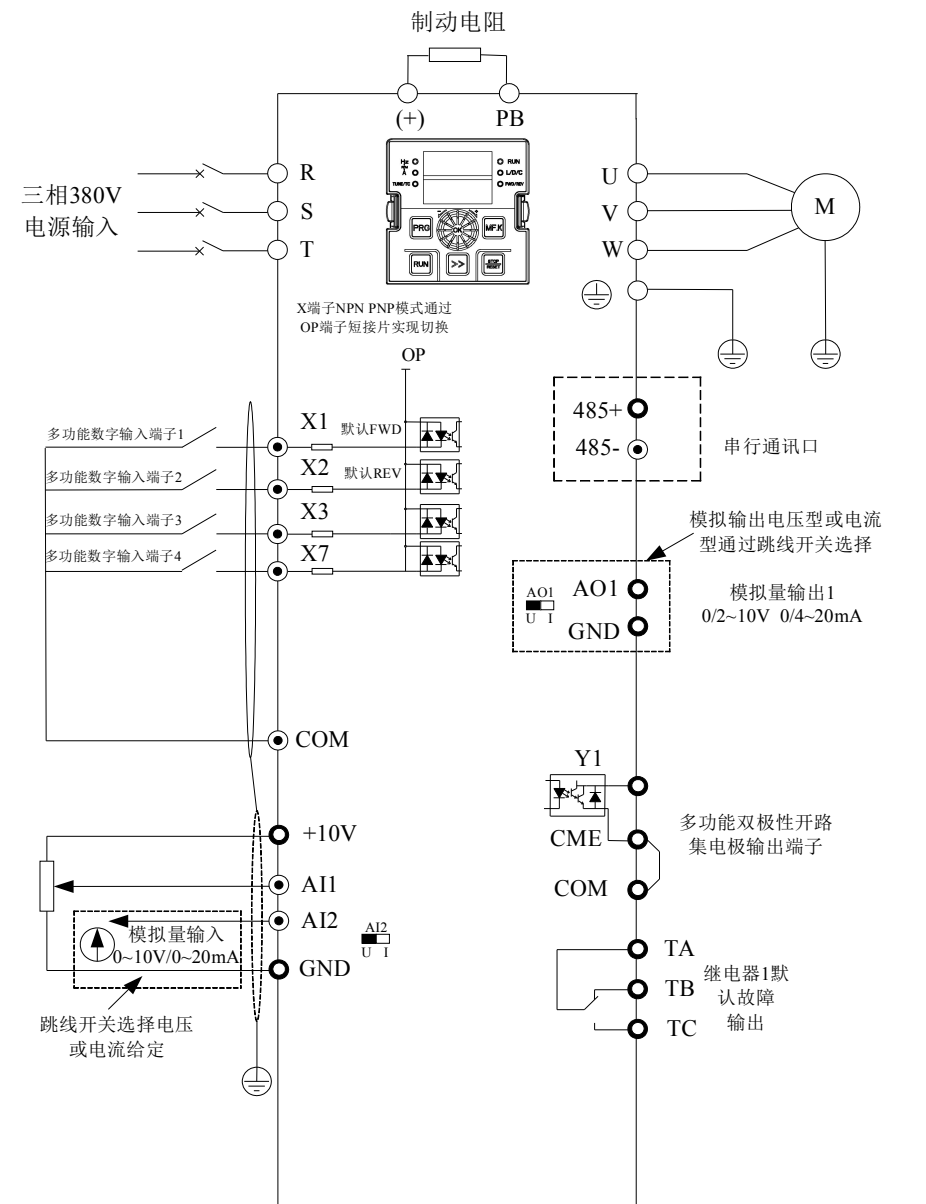
图3-1. 三相380V 2.2kW (4T:380V) 及单相220V (2S) 2.2kW(输入接L N或R T)以下变频器接线图 备注：数字输入端子X跳线开关出厂默认（OP端子连接24V端子）NPN模式（即X短接COM有效），PNP模式为选配功能，三相380V 2.2 kW 及单相220V 1.5 kW 以下如需选配PNP模式，订货时请说明。AI2,A01跳线开关出厂默认电压模式。
