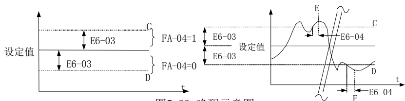
图5-33. 唤醒示意图
