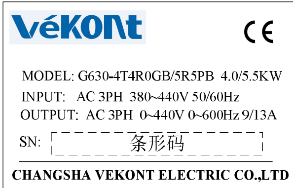
图2-2. 铭牌
