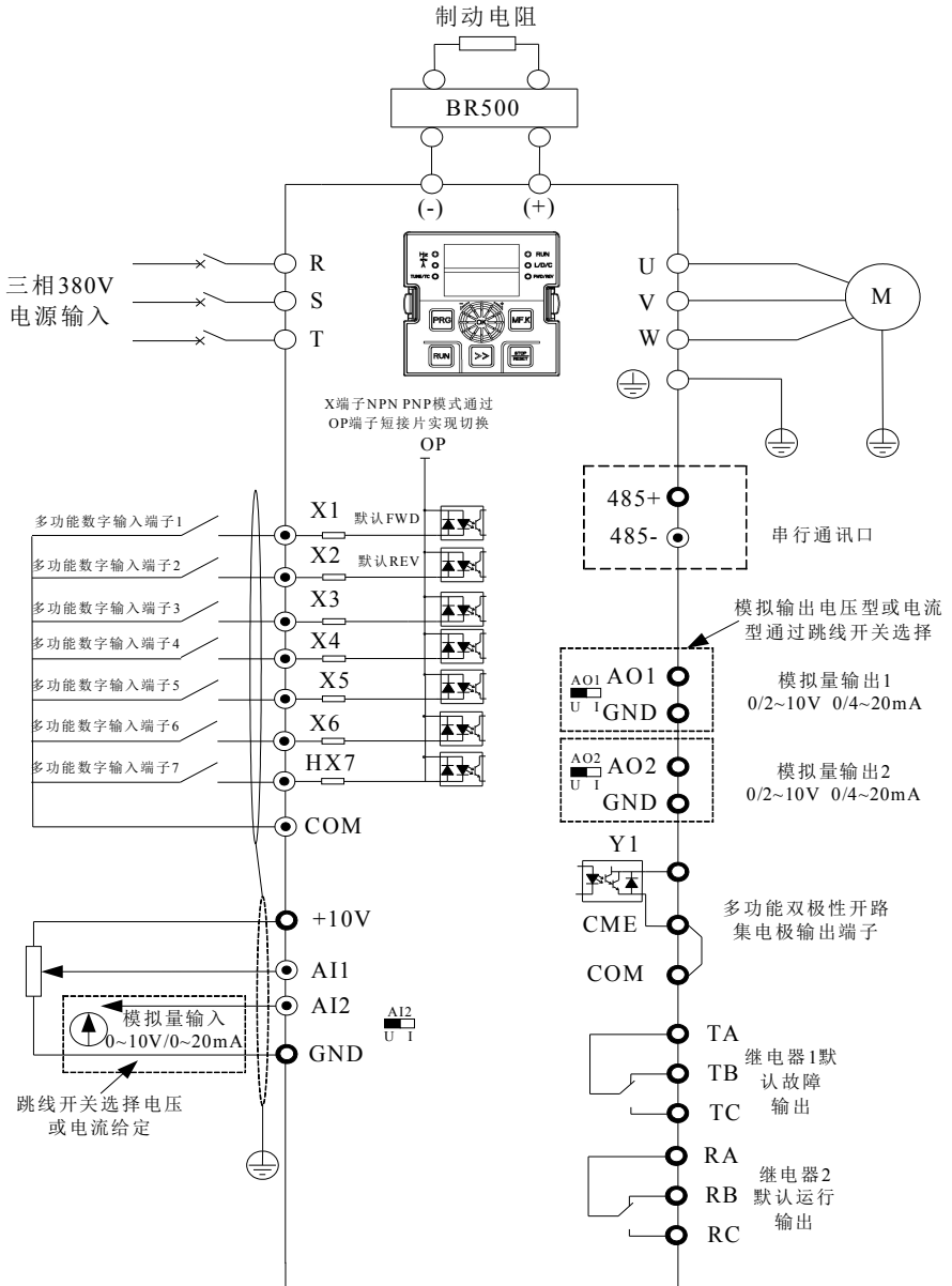
图 3-3. 三相 380V 37 ~ 75 kW (4T:380V) 变频器不带制动单元元功能接线图
