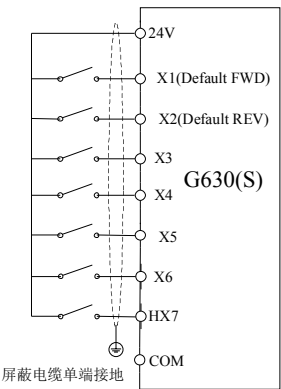
图 3-11. 四种不同模式下数字输入端子接线图
