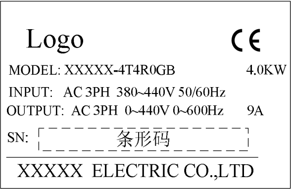
图 2-2. 铭牌
