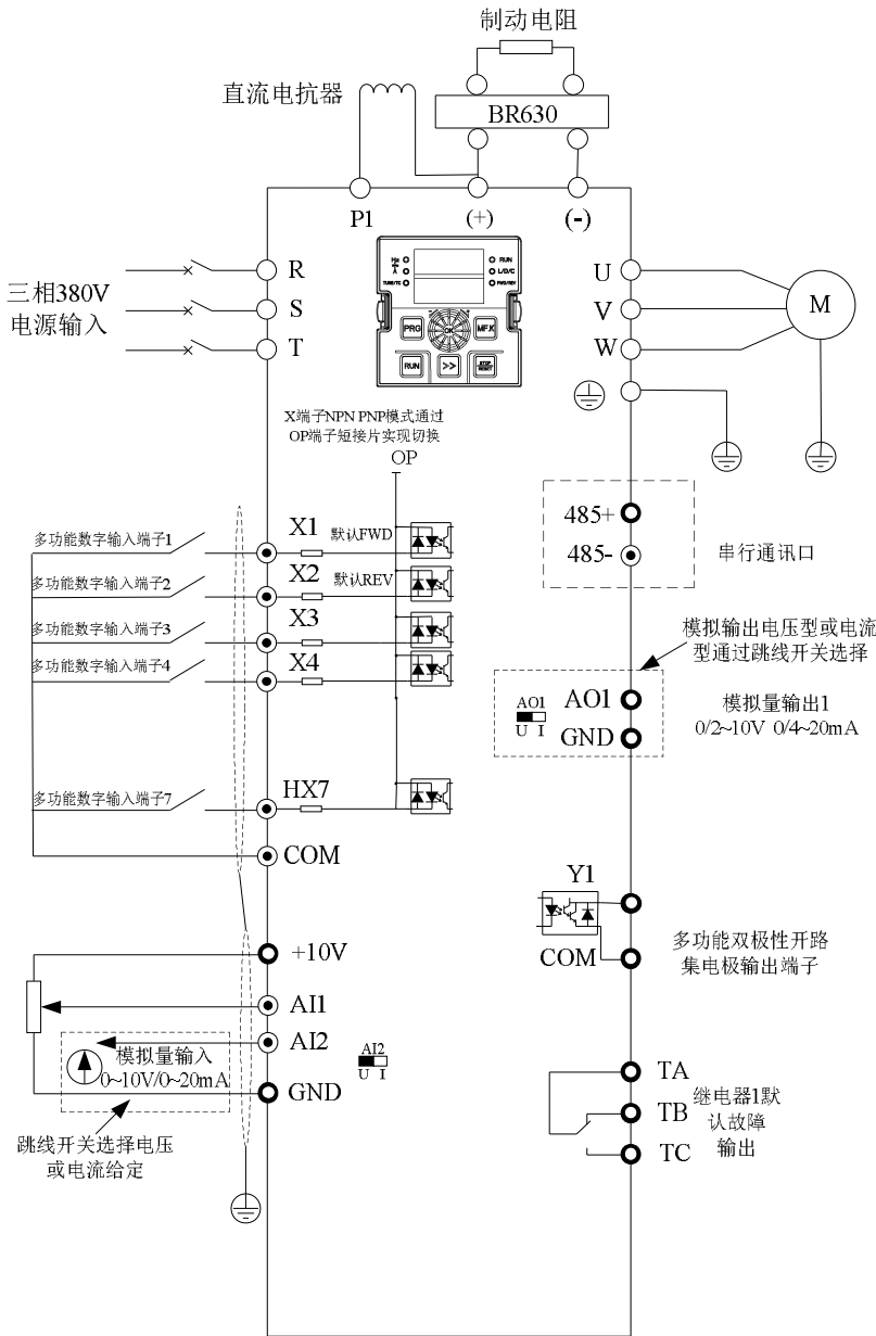
图 3-4. 三相 380V 132kW（4T:380V）及以上三相变频器接线图
