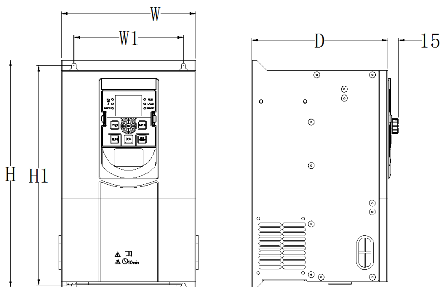
图 2-5. 380V (4T) 18.5~220kW 钣金机箱外形尺寸及安装尺寸示意图
