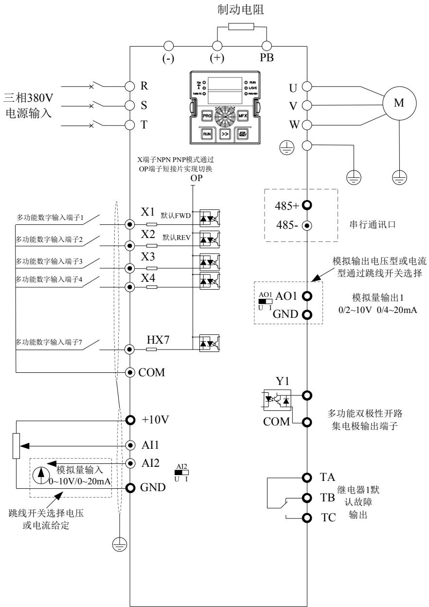
图 3-2. 三相 380V 4.0~ 37kW (4T:380V) 及单相 220V (2S) 4.0~ 5.5kW 以下(输入接 R T)变频器 接线图
