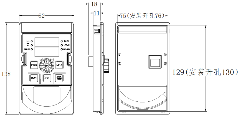
图 2-8.1 380V（4T）4.0kW以上外引键盘带托盘安装尺寸图
