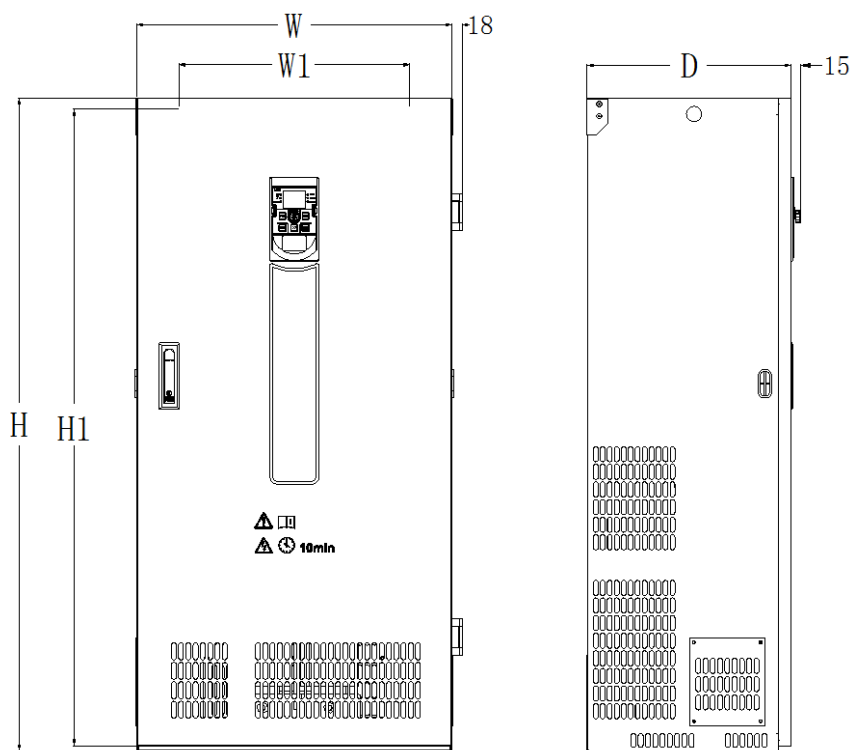
图 2-6. 380V 250kW 以上变频器外型尺寸及安装尺寸示意图
