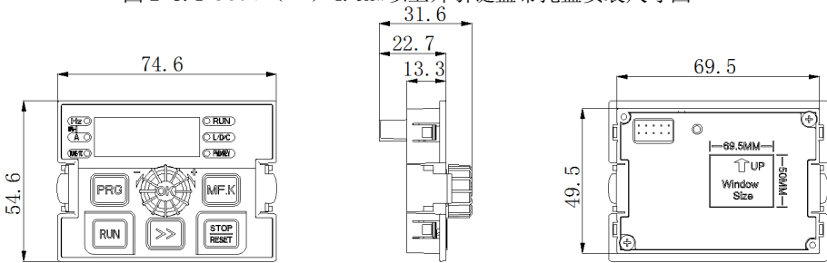
图 2-8.2 380V（4T）2.2kW以下外引键盘不带托盘安装尺寸图
