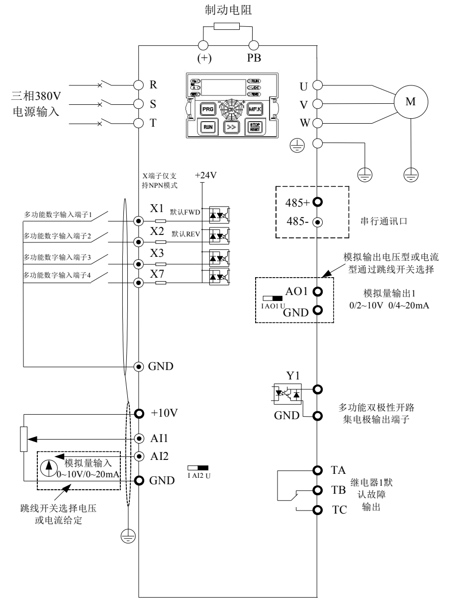
图3-1. 三相380V 2.2kW (4T:380V) 及单相220V (2S) 2.2kW(输入接L N或R T)以下变频器接线图 备注: 数字输入端子 X 2.2kW 出厂默认(OP 端子连接 24V 端子)NPN 模式(即 X 短接 GND 有效)。AI2, AO1 跳线开关出厂默认电压模式。
