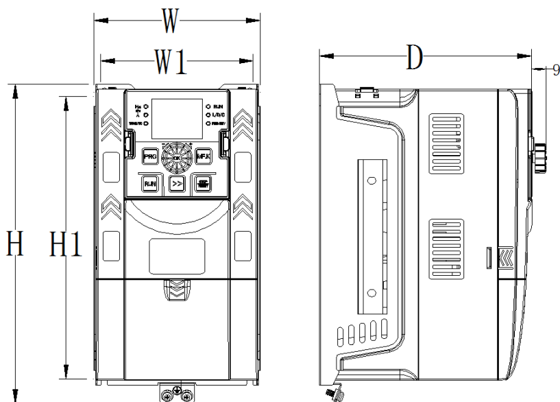
图 2-4. 380V (4T) 15kW 以下塑胶外形尺寸及安装尺寸示意图
