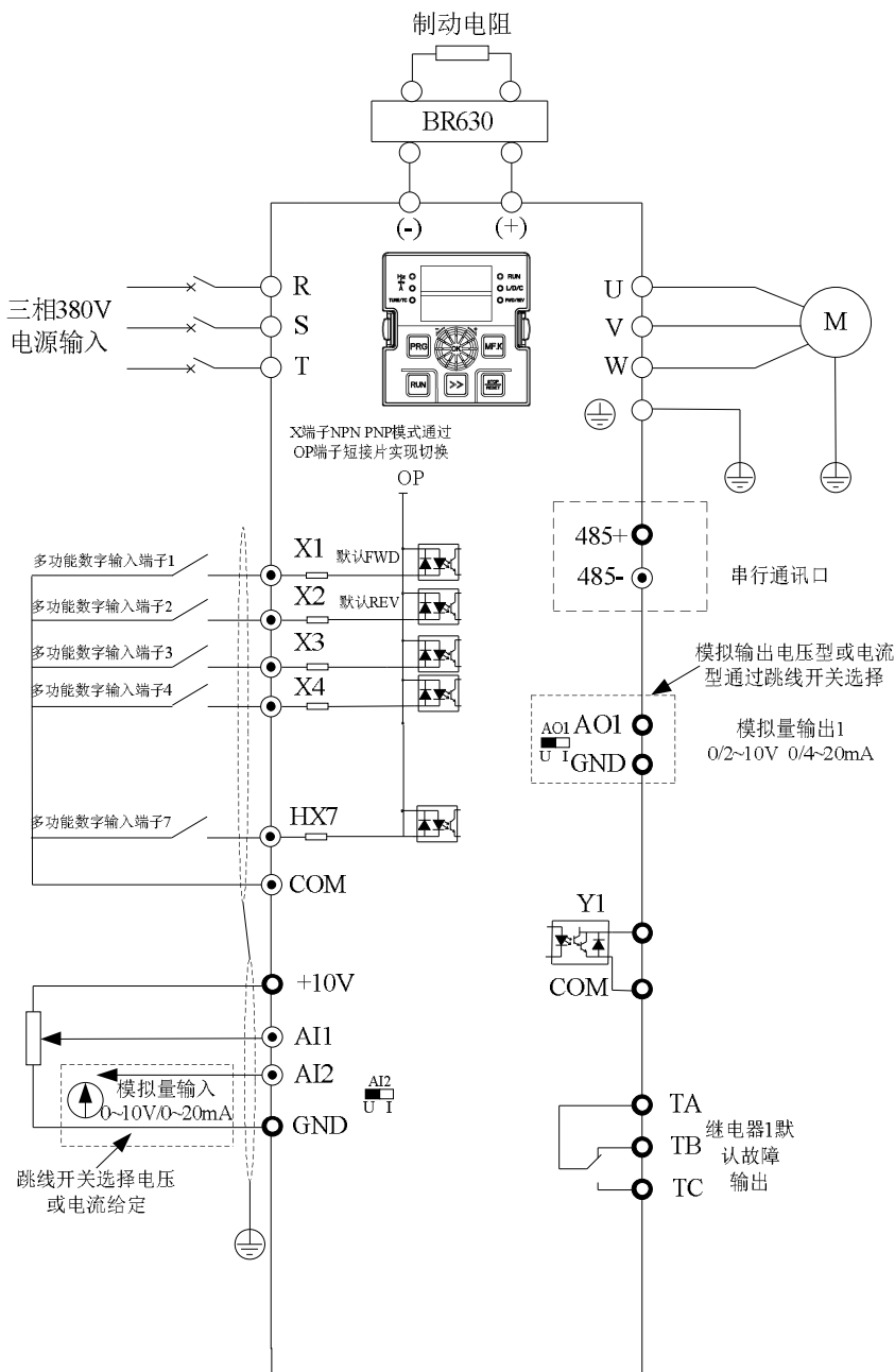
图 3-3. 三相 380V 55 ~ 110 kW (4T:380V) 变频器不带制动单元功能接线图
