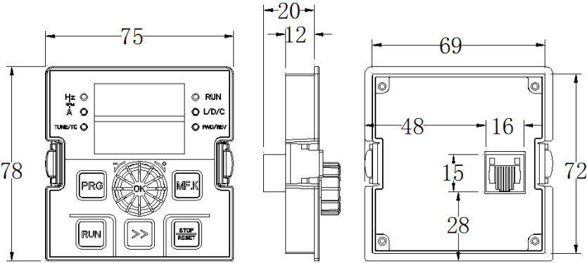
图 2-9.1 380V（4T）4.0kW以上外引键盘不带托盘安装尺寸图
