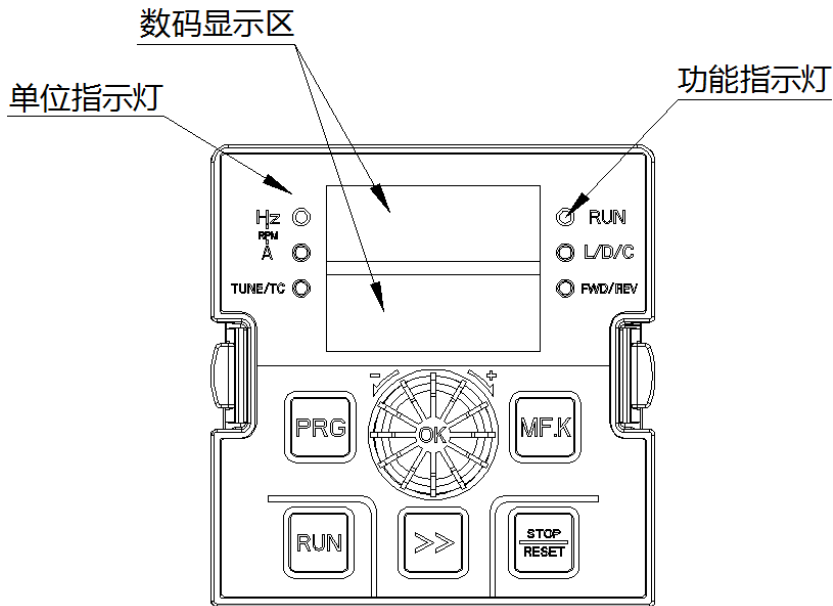
图 4-1. 操作面板示意图 1(标配单行显示LED键盘 1，选配双行显示 630-LED键盘 1)
