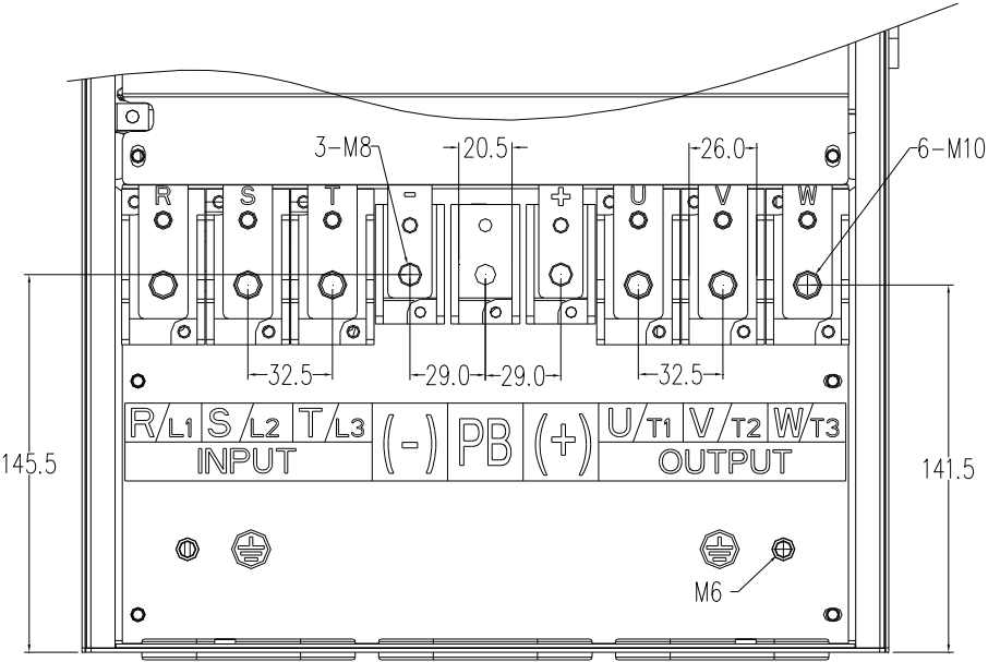
三相 380V（4T）037~045kW(G 型机)主回路接线端子尺寸图
