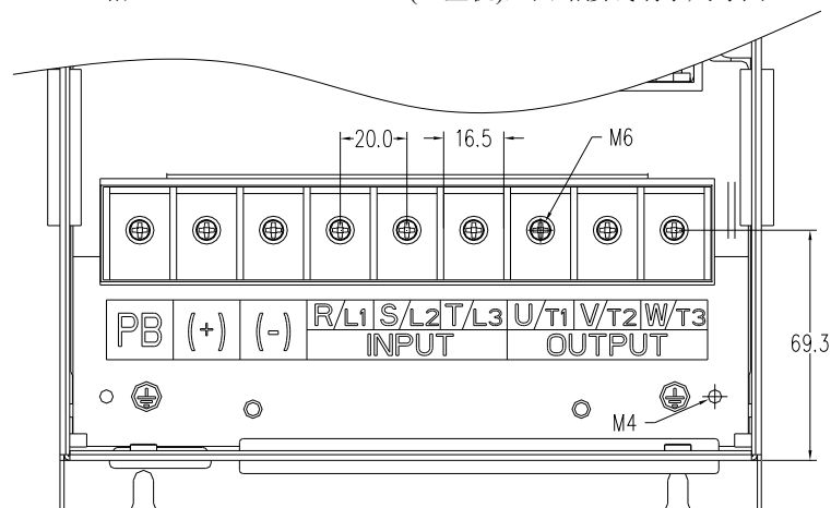
三相 380V (4T) 030kW(G 型机)主回路接线端子尺寸图
