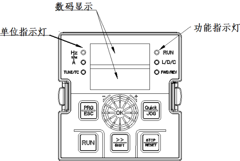
图4-1. 操作面板示意图I(标准配置LED键盘I)
