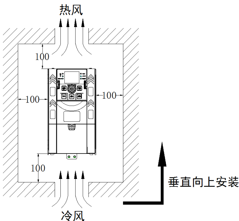
图3-1. 单体安装图
