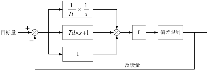
图5-23. 过程PID原理框图
