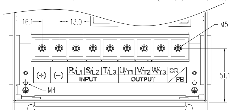
三相 380V (4T) 7.5~11kW 及单相 220V (2S) 4.0~5.5kW (G 型机)主回路接线端子尺寸图
