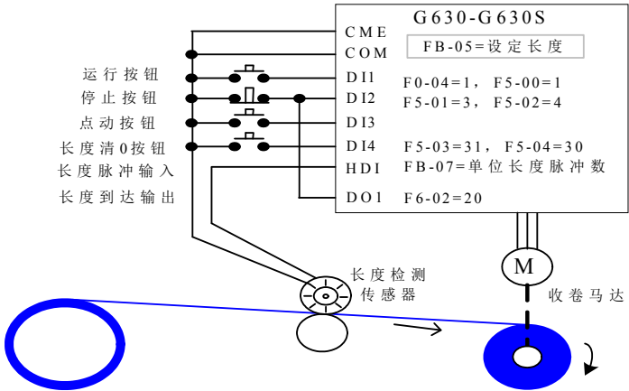
图 4-24. 定长控制功能常见应用举例
