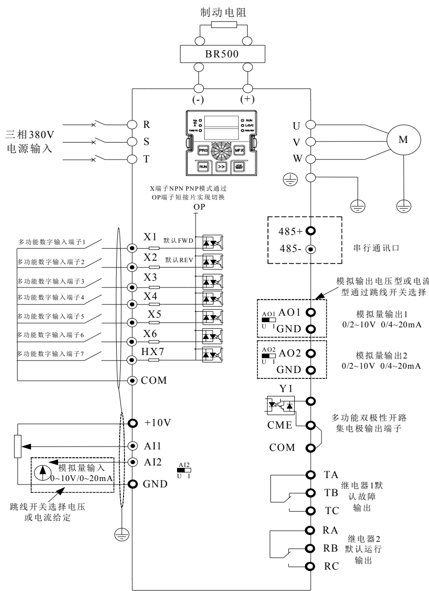
图 3-3. 三相 380V 37 ~ 75 kW (4T:380V) 变频器不带制动单元功能接线图
