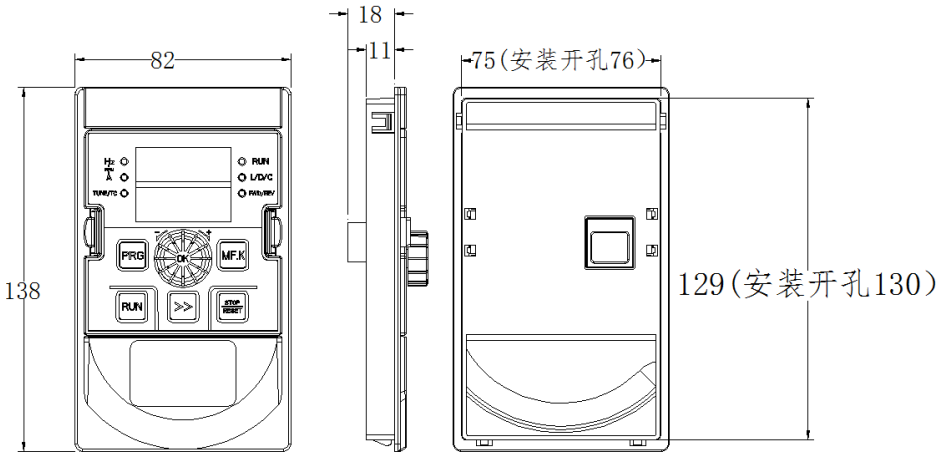
图 2-8. 1 外引键盘带托盘安装尺寸图
