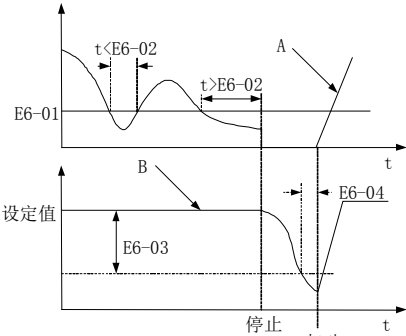
图5-32. 休眠过程频率图
