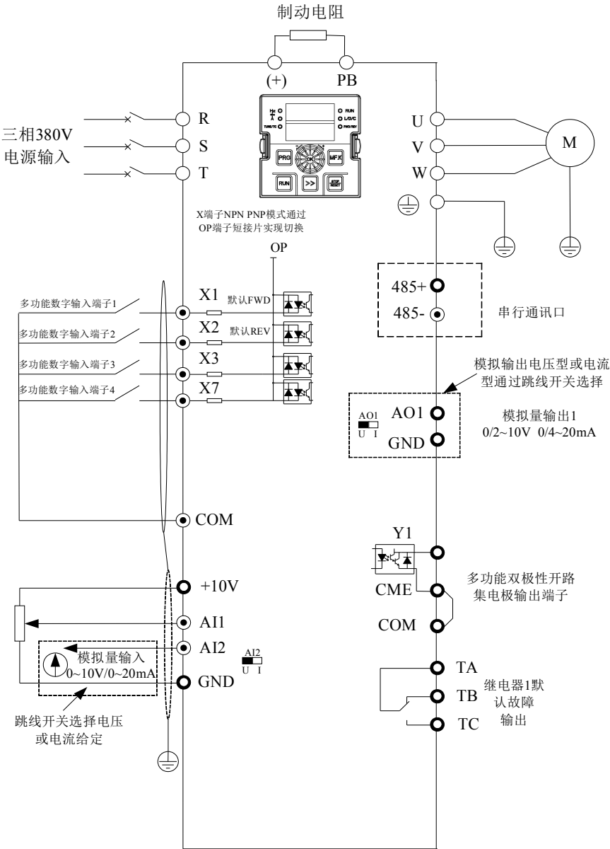
图3-1. 三相380V 2.2kW (4T:380V) 及单相220V (2S) 2.2kW(输入接L N或R T)以下变频器接线图
