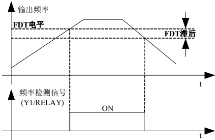
图 5-15. FDT 电平示意图
