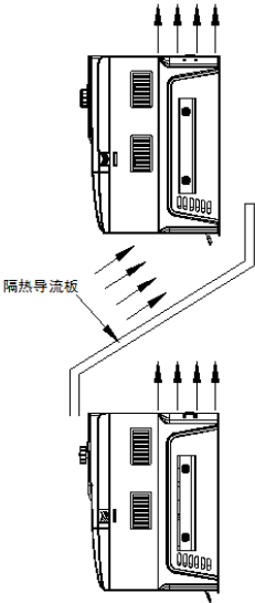
图3-2. 630/630S变频器安装示意图
