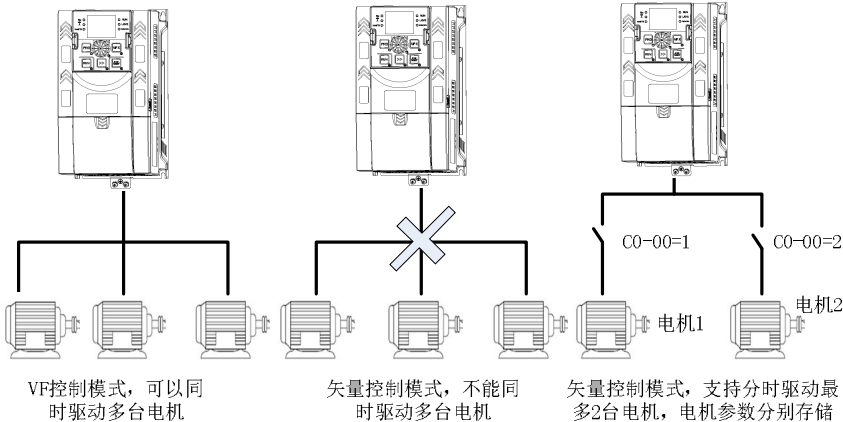
图 4-26. 多组电机的切换
