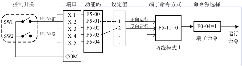
图4-8. 端子控制启停示意图
