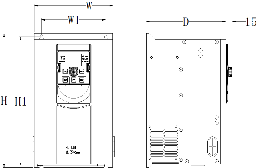
图 2-5. 15~200KW 钣金机箱外形尺寸及安装尺寸示意图
