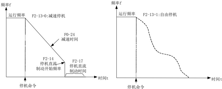
图4-13. 停机示意图
