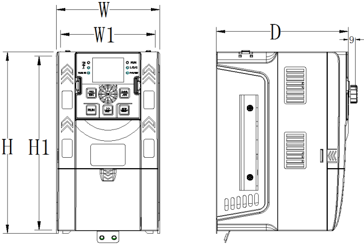
图 2-4. 11KW 以下塑胶外形尺寸及安装尺寸示意图
