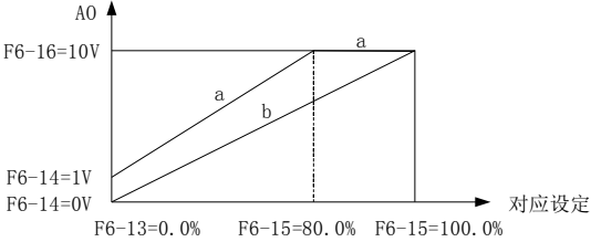
图4-29. F0输出示意图
