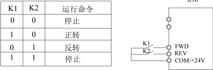
图 5-7. 两线式运转模式 1
