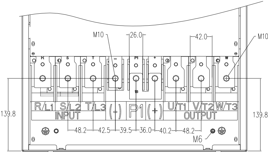
三相 380V (4T) 093~110kW(G 型机)主回路接线端子尺寸图
