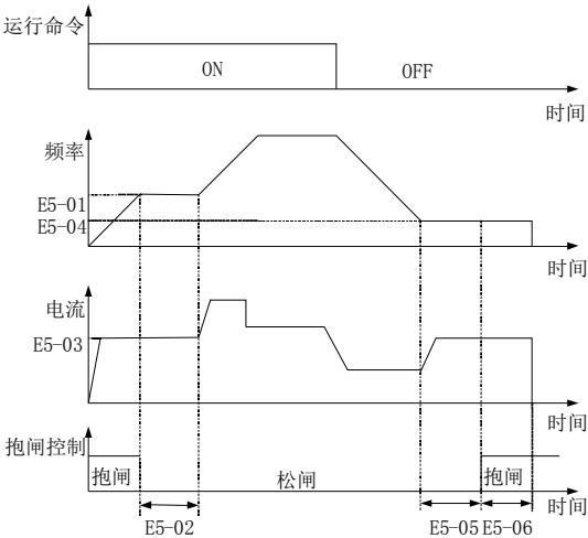
图5-31. 抱闸控制过程图
