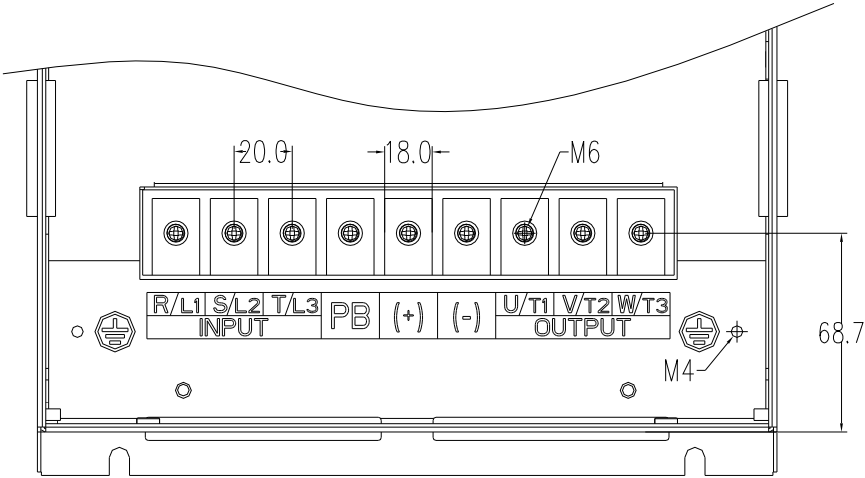
三相 380V（4T）037~045kW(G 型机)主回路接线端子尺寸图
