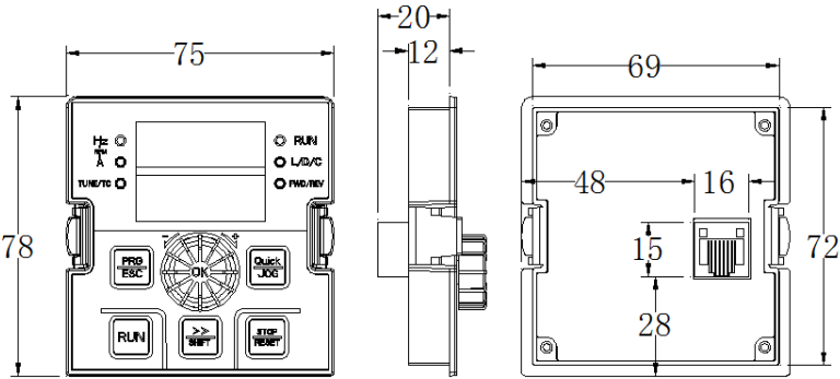
图 2-9.1 外引键盘不带托盘安装尺寸图
