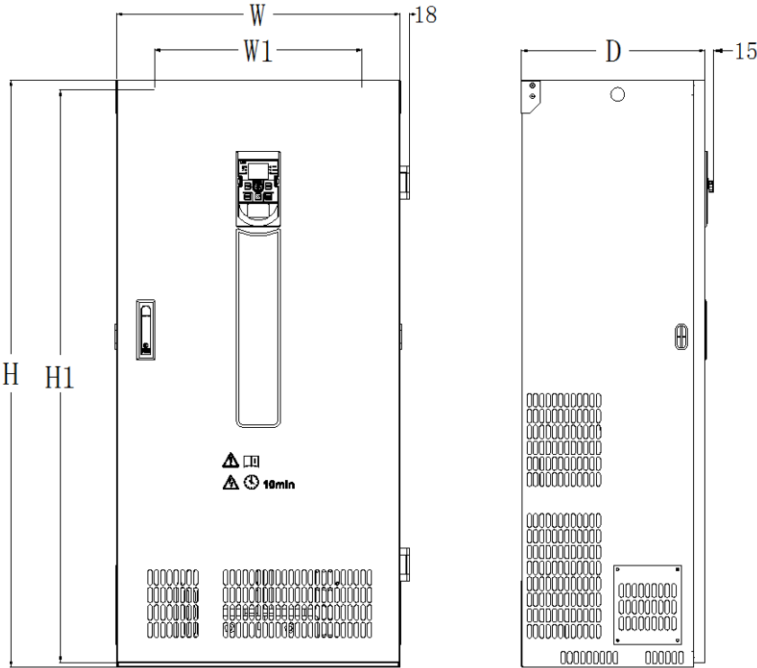
图 2-6. 160KW 以上变频器外型尺寸及安装尺寸示意图 表 2-2 630/630S 外形尺寸及安装孔位尺寸
