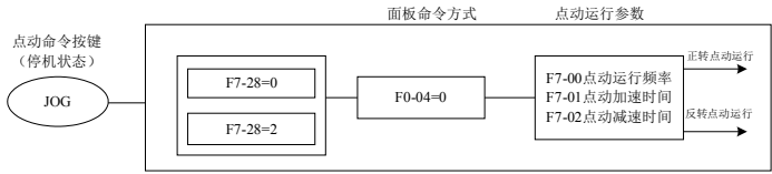
图4-15. 点动参数设定示意图
